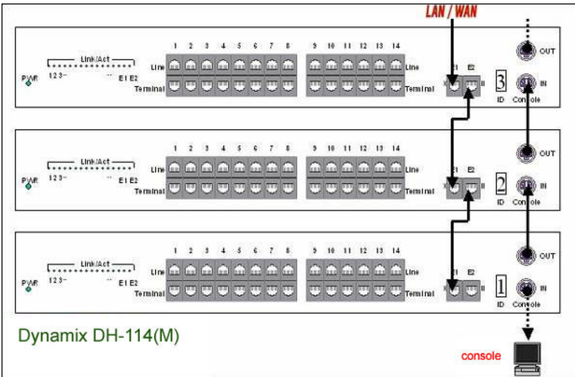
Figure 2 Cabling of more DYNAMIX DH - 114/DYNAMIX DH - 114 M
