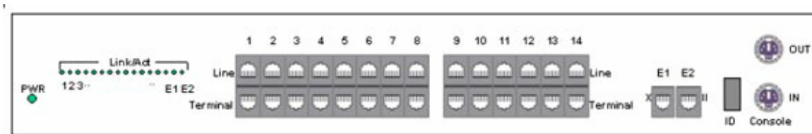
Figure 1 Front panel of DYNAMIX DH - 114/DYNAMIX DH - 114 M
